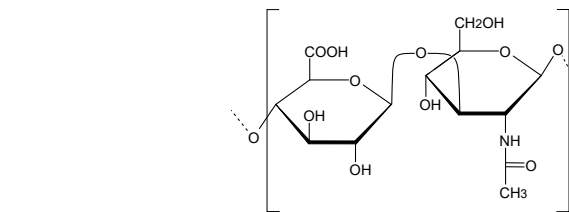
Exemple d'un GAG : l'acide hyaluronique
